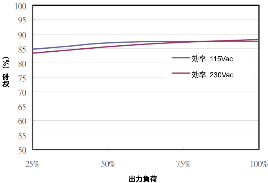
図 1 効率と出力負荷の比較
